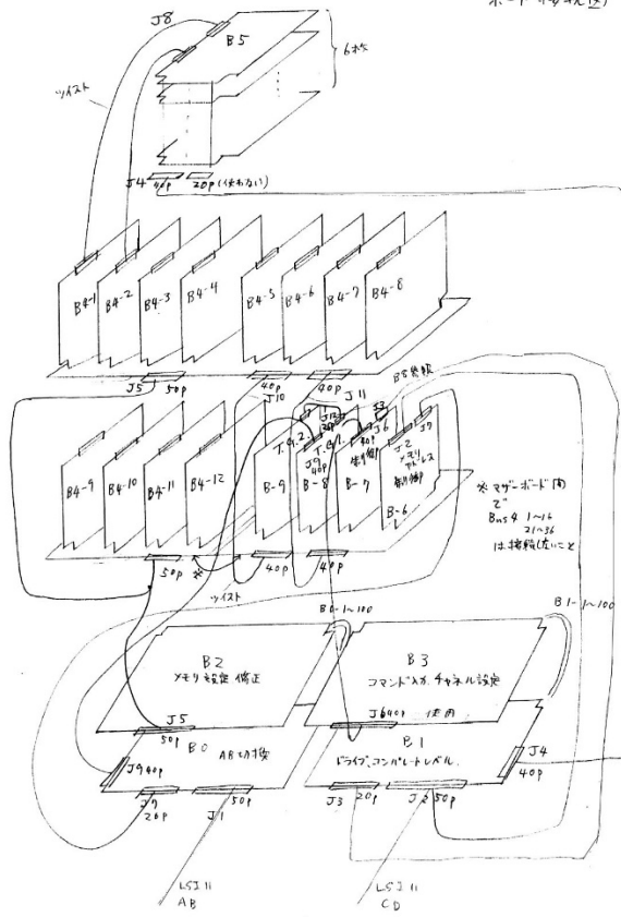
ポート回路図
