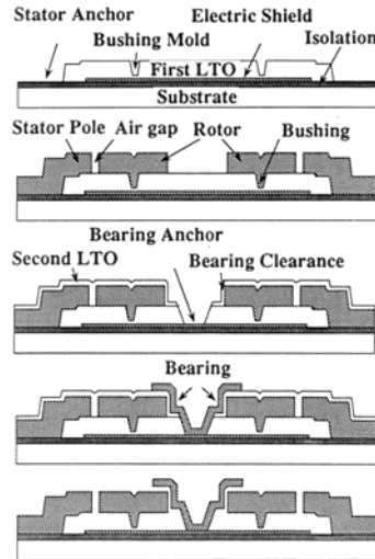
Electrostatic micro motor (MIT USA)
