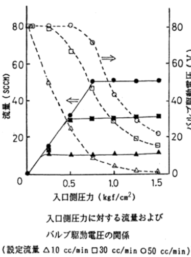
サーマルマスフローセンサ + マイクロバルブ 集積化マスフローコントローラ
