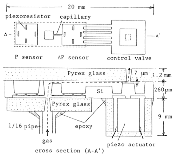
差圧式マスフローセンサ + マイクロバルブ
