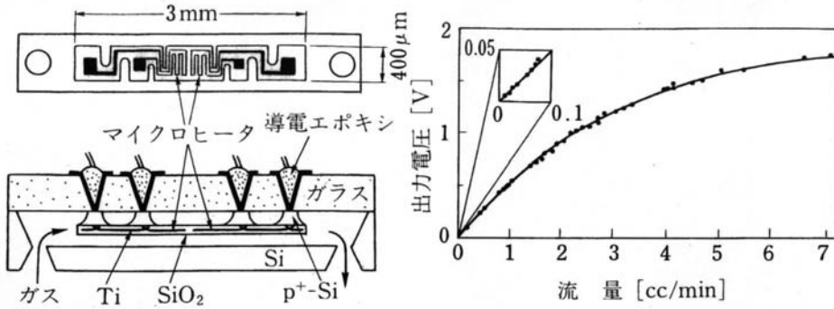
サーマルマスフローセンサ
