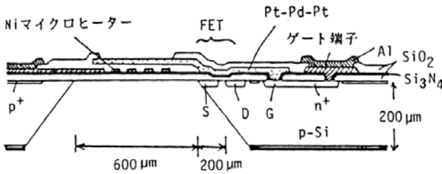
延長ゲート Pd ゲート FET (東北大 - リンシェピン工科大(スウェーデン))
