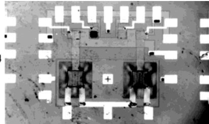
延長ゲート Pd ゲート FET (東北大 - リンシェピン工科大(スウェーデン))
