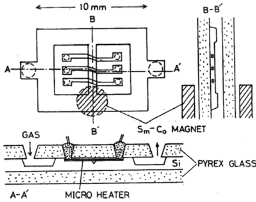
磁気式酸素センサ
