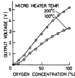
磁気式酸素センサ
