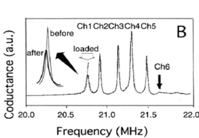
水晶の Deep RIE によるマルチ QCM
