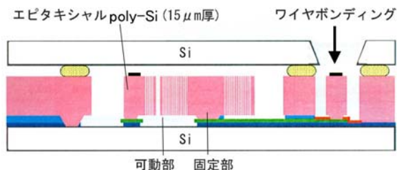
ST マイクロエレクトロニクス社の加速度センサ
