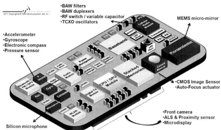
モバイル機器内の MEMS (Yole Development)
