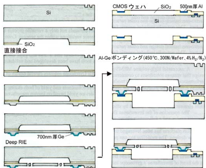
Invensense 社のジャイロ
