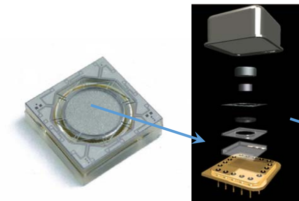
電磁式シリコンリング式ジャイロ
