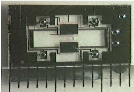
Deep RIE で製作した電磁駆動静電容量検出振動ジャイロ
