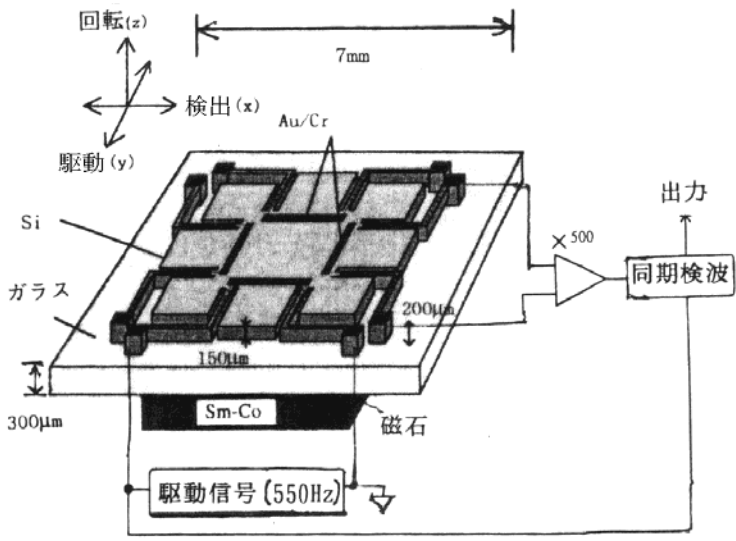
Z 軸用電磁駆動電磁(誘導起電力)検出振動ジャイロ
