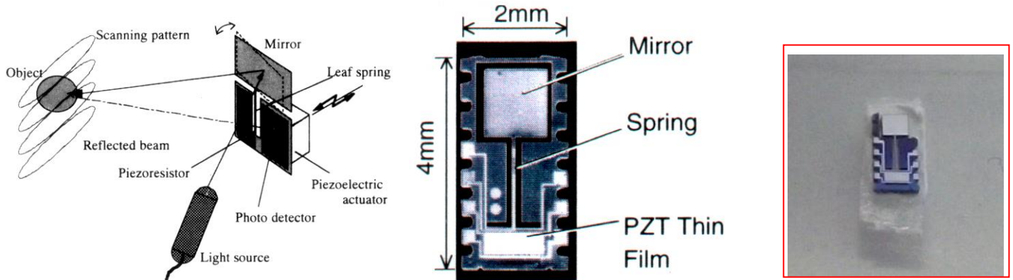
圧電 2 軸光スキャナ (オムロン)
