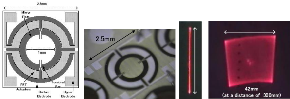
レーザープロジェクタ用圧電薄膜 2 軸光スキャナ
