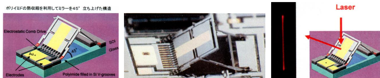
バーコードリーダ用静電光スキャナ (東北大 - オプトエレクトロニクス)
