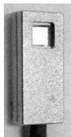
シリコンマイクロホン (NHK) (T. Tajima, N. Saito, M. Esashi et al., Microelectronic Engineering, 67-68 (2003) 508)
