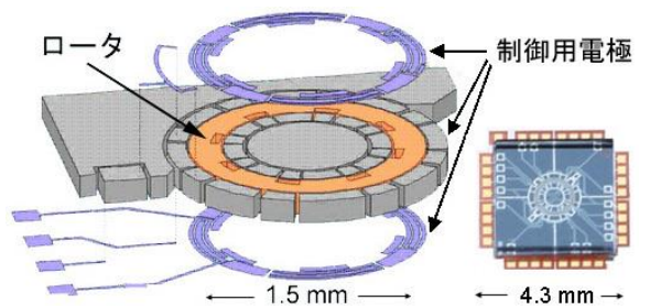
静電浮上回転ジャイロ (東京計器株)
