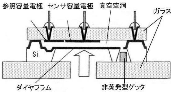
シリコン容量型真空計 (宮下治三、北村恭志、アネルバ技報, 11 (2005) 37)
