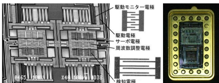
ヨーレート・加速度センサ (トヨタ自動車株)
