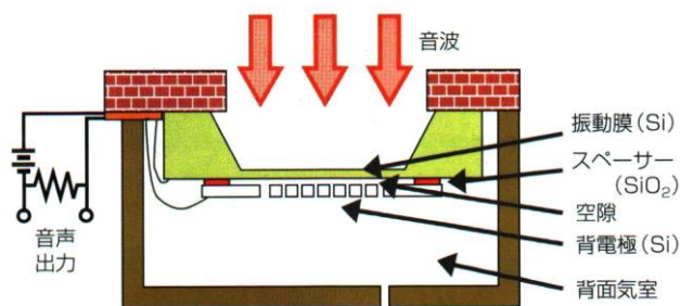
シリコンマイクロホン (NHK) (T. Tajima, N. Saito, M. Esashi et al., Microelectronic Engineering, 67-68 (2003) 508)
