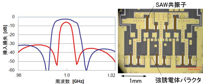
SAW デバイスへの強誘電体可変容量素子の選択転写による可変帯域フィルタ
