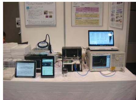
SAW デバイスへの強誘電体可変容量素子の選択転写による可変帯域フィルタ
