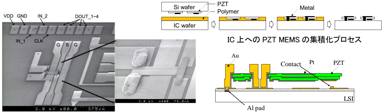
0.35 μm CMOS 上に作製した PZT 圧電駆動 MEMS スイッチ (Matsuo et al., IEEE MEMS 2012, pp. 1153-1156)
