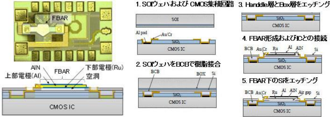
LSI 上に製作した FBAR (film bulk acoustic resonator) (Kochhar et. al, 2012 IEEE Internl. Ultrasonic Symp. (2012) 1047)
