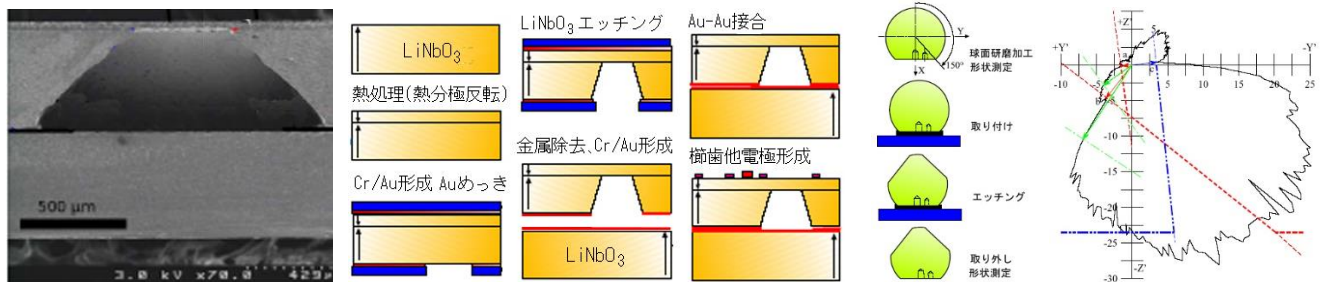
LiNbO 3 ダイアフラム、および熱分極反転と結晶異方性エッチングによる製作法 LiNbO 3 の結晶異方性エッチング
