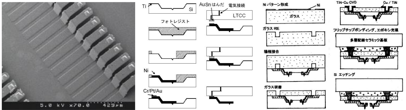
LSI ウェハ検査用プローブカード (S.-H. Choe et. al., IEEE Internl. Test Conf. 2007 (2007))
