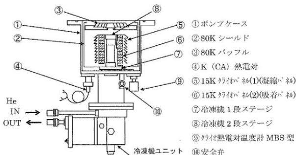
クライオポンプの構造と写真
