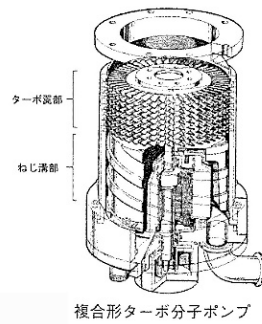
ターボ分子ポンプ
