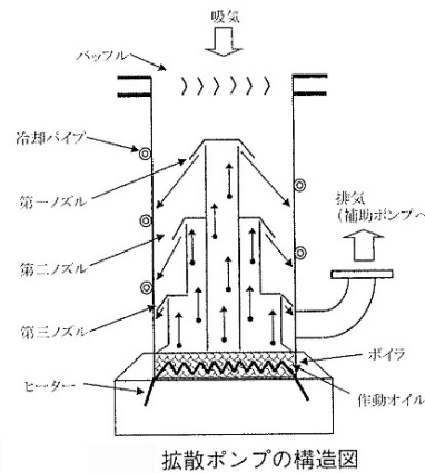
(油)拡散ポンプの原理・構造・写真（展示(ガラス製 熊野勝文氏製作)）
