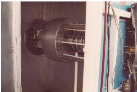
イオン注入装置（アクセレータ社 200kV 前段加速型）
