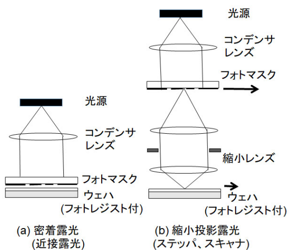
露光装置の原理
