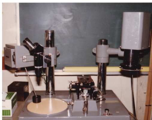
片面密着露光装置とそれを改造した両面密着露光装置
