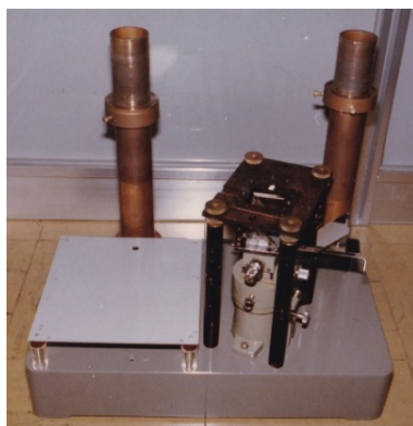
片面密着露光装置とそれを改造した両面密着露光装置
