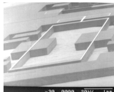
ドライエッチング(Si 反応性イオンエッチング(DRIE))
