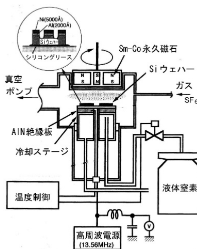
ドライエッチング(Si 反応性イオンエッチング(DRIE))
