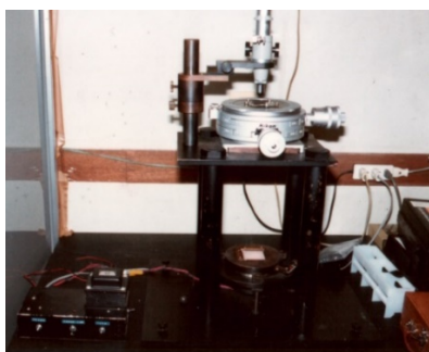
1/10 縮小カメラ (乾板上に並べて写す)
