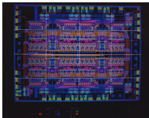
レイアウト図 (グラフィックエディタは Fortran で作成)
