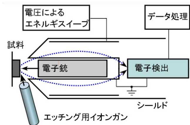
同軸電子エネルギーアナライザ(CMA)(展示)を用いたオージェ電子分光装置
