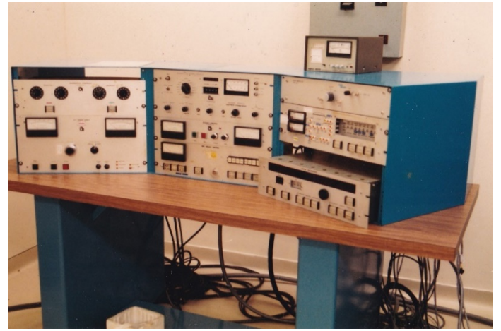
イオン注入装置 (アクセレータ社 200MP 中古)
