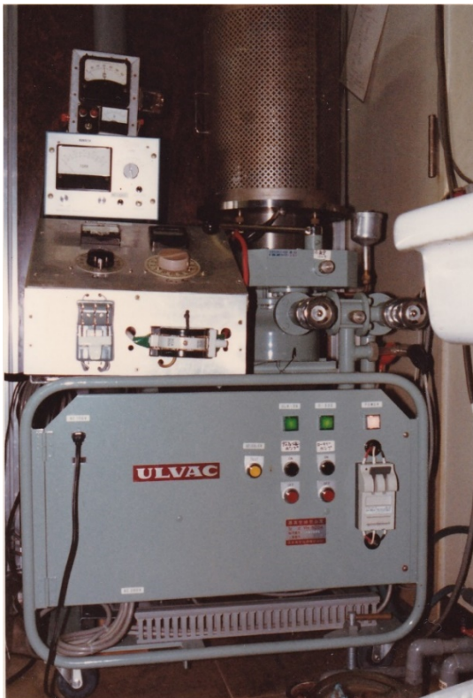
Al, Cr-Cu-Au 蒸着装置
