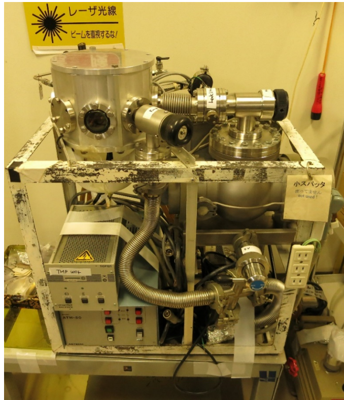
マグネトロンスパッタ堆積装置
