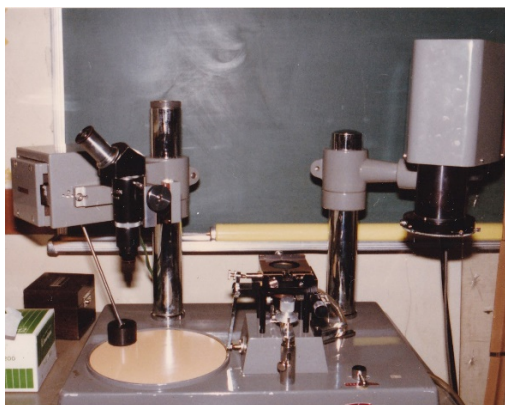
マスクアライナ(左)と両面露光用ステージ(右)
