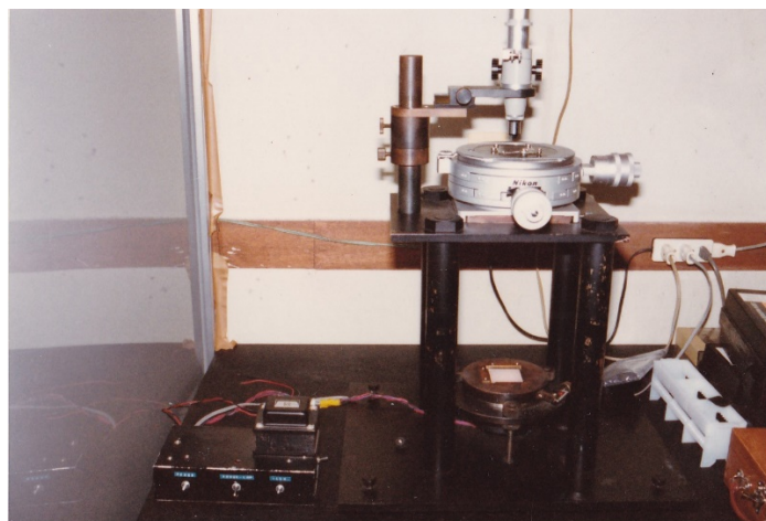
フォトリピータ
