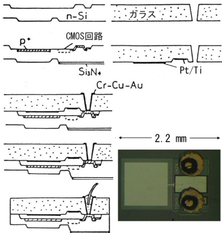
ウェハレベルパッケージングによる集積化容量型圧力センサ (松本佳宣、江刺正喜：絶対圧用集積化容量形圧力センサ，電子情報通信学会論文誌 C-II, J75-C-II, 8 (1992) 451-461)
