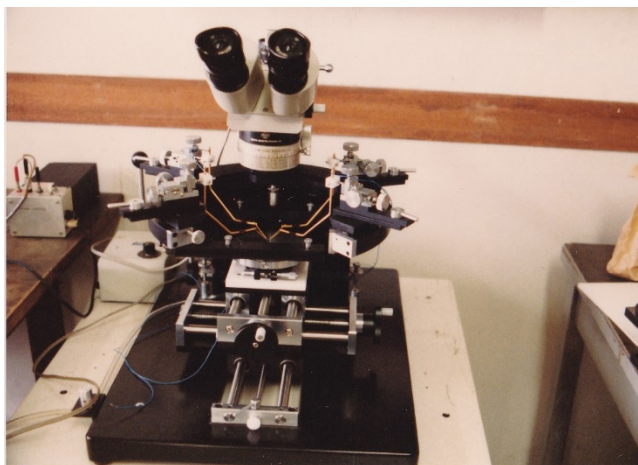
ウェハプローバ
