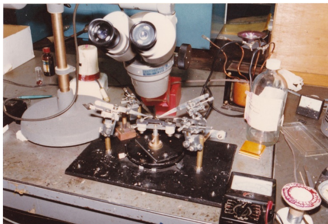
微小はんだ付け(導電性接着)装置
