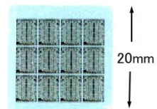
20mm 角ウェハ上に製作した CMOS LSI
