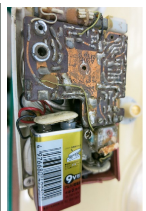
トランジスタラジオ(ソニー TRW-621)(1960) (時計はタイマーとして使用可) [2]
