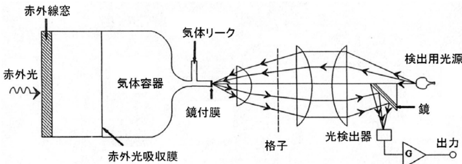
ゴーレーセル (気体の熱膨張による赤外線光の検出)
