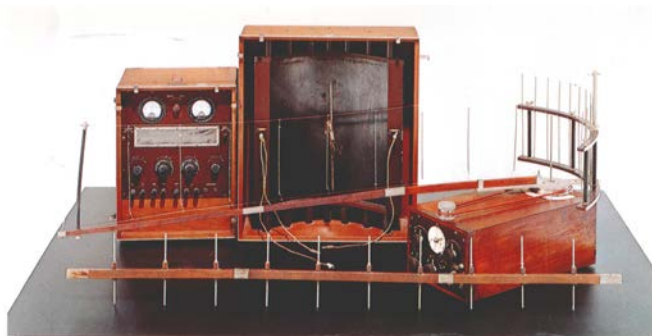
八木アンテナ (1928) (「東北大学」編集委員会編、「東北大学」 2007/8/1)
