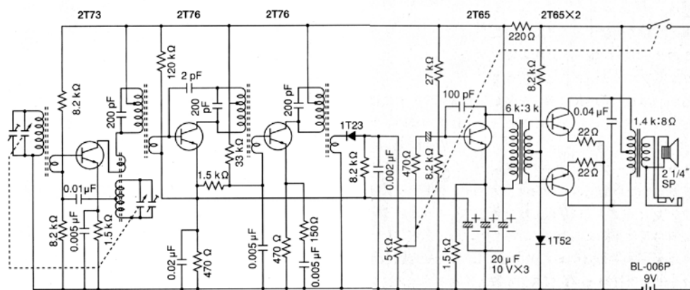
トランジスタラジオ(1955)[2] (相良岩男, 20世紀エレクトロニクスの歩み:日経エレクトロニクス(1996))
