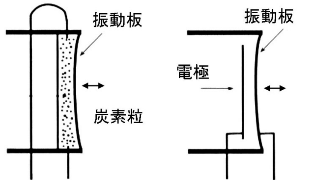
炭素粒マイクロホン コンデンサマイクロホン エジソン(1877)
