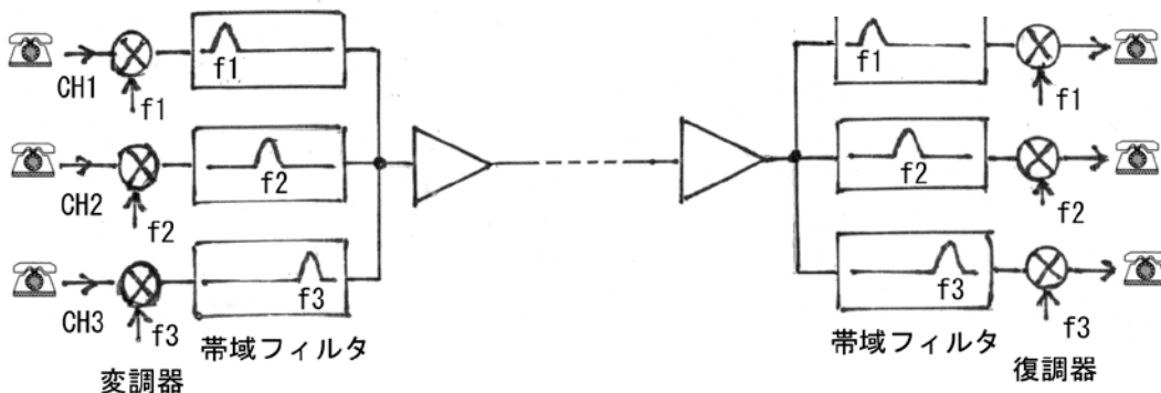
(c) 無装荷ケーブルによる多重通信
