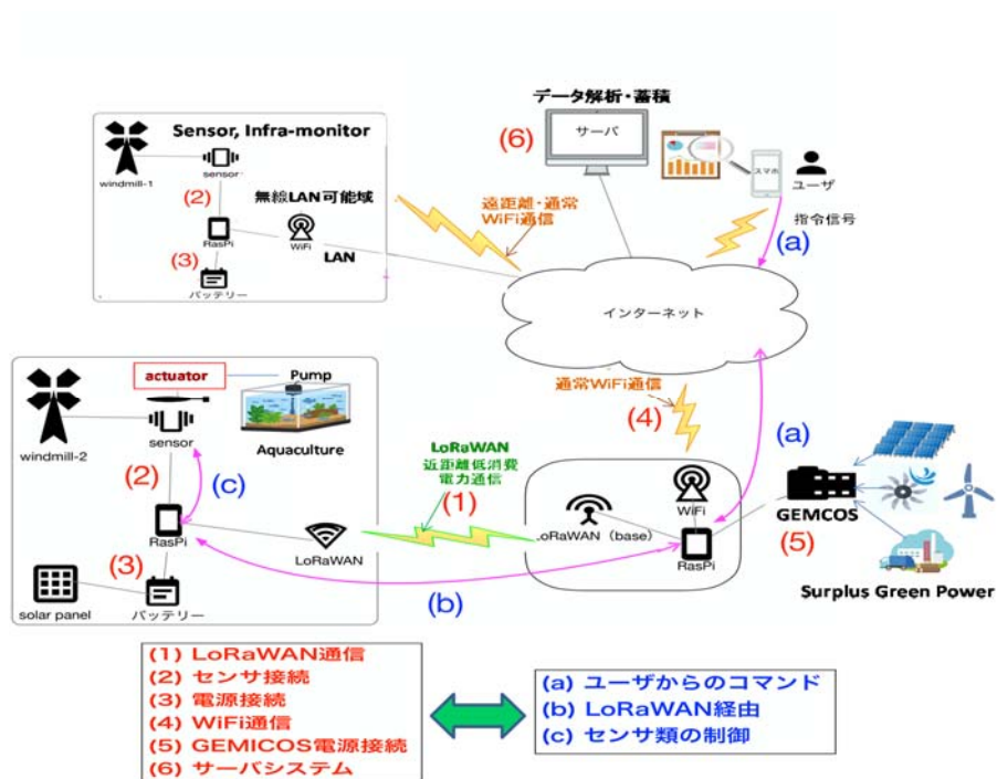
図7 開発した低消費電力近～中距離無線 LoRaWAN によるグリーンエネルギー開発地点での2次産業機器操作・診断に向けての「GEMCOS-IoT双方向ACTIVE制御システム」の構成図
