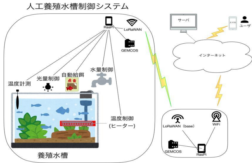
図8 双方向IoTセンサネットワークを用いた、人工養殖水槽での制御システム図 =水槽の温度制御に、外部水源からのポンプ流速の変化や、自動餌やりシステムが可能=
